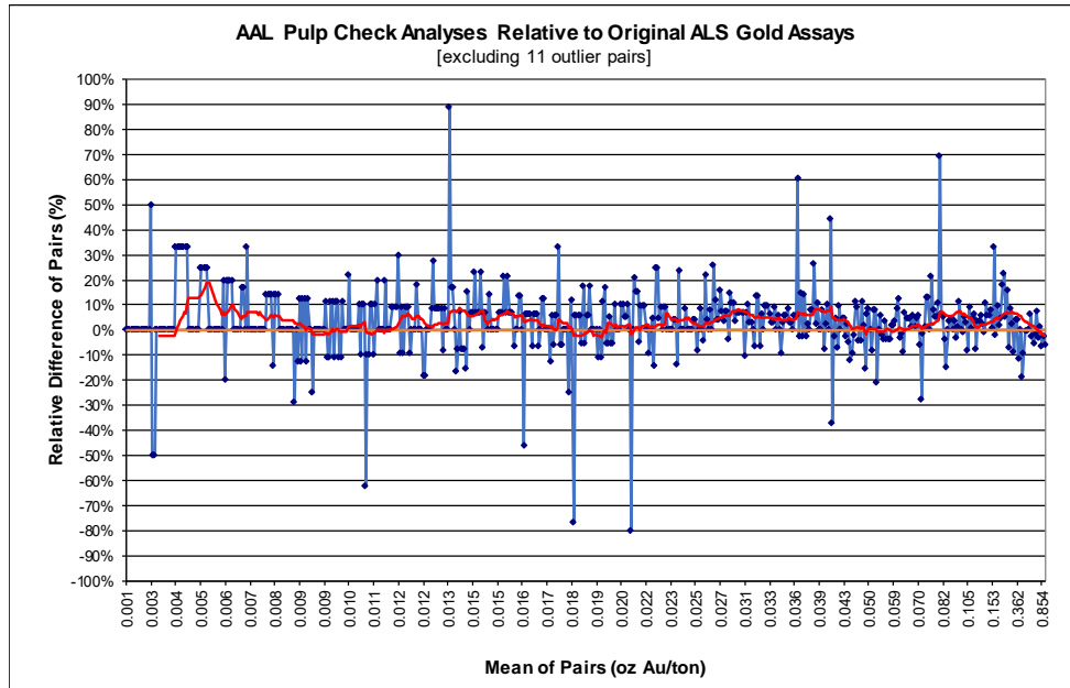
Figure 11-10: AAL Pulp Checks of ALS Original Gold Analyses
