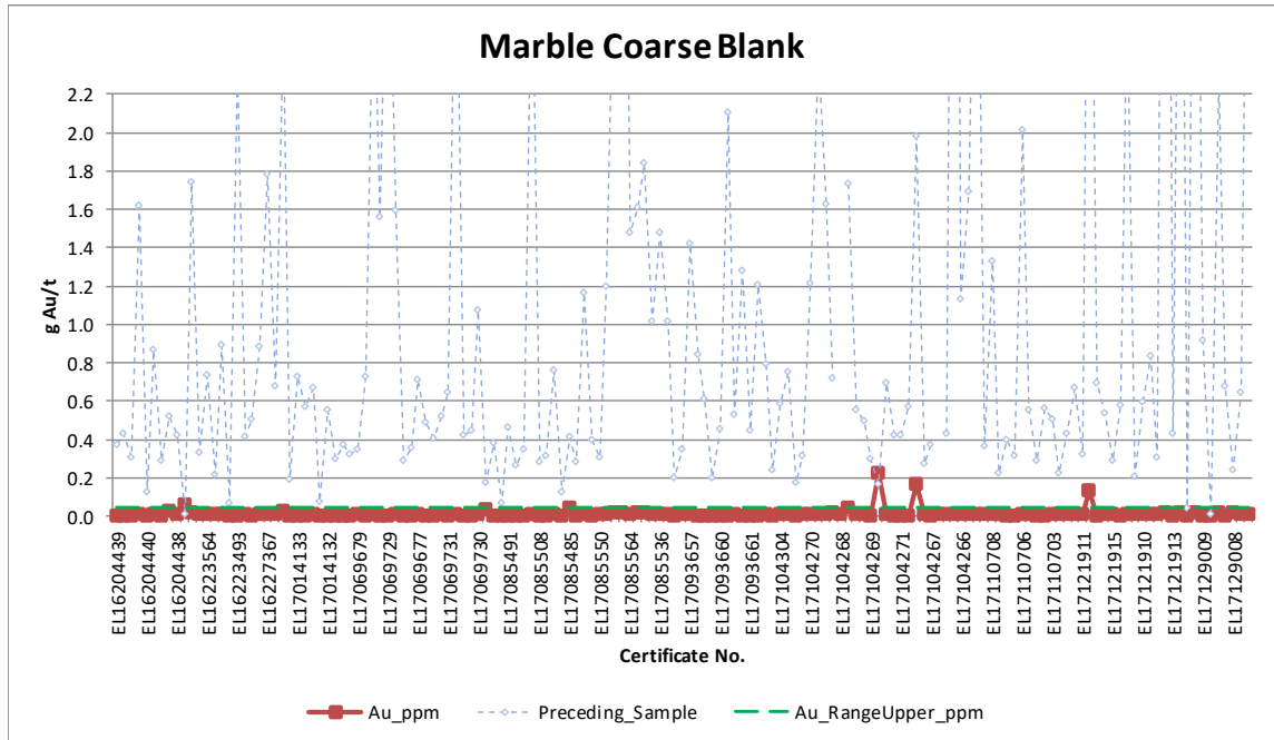
Figure 11-11: Chart of ALS Analyses of Coarse Blanks - Paramount
