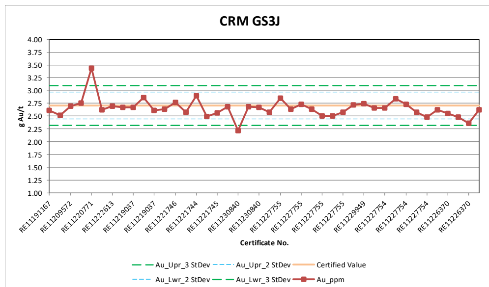
Figure 11-8: Chart of ALS Analyses of CRM CDN-GS-3J
