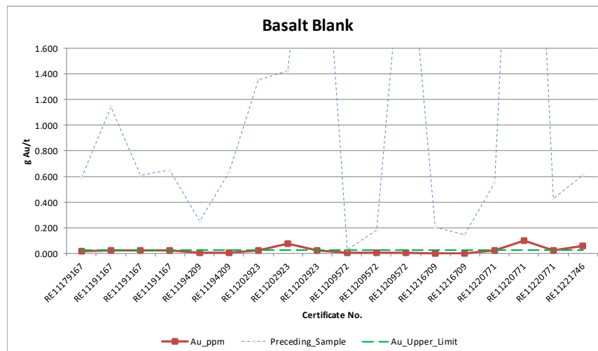
Figure 11-9: Chart of ALS Analyses of Coarse Blanks - Calico
