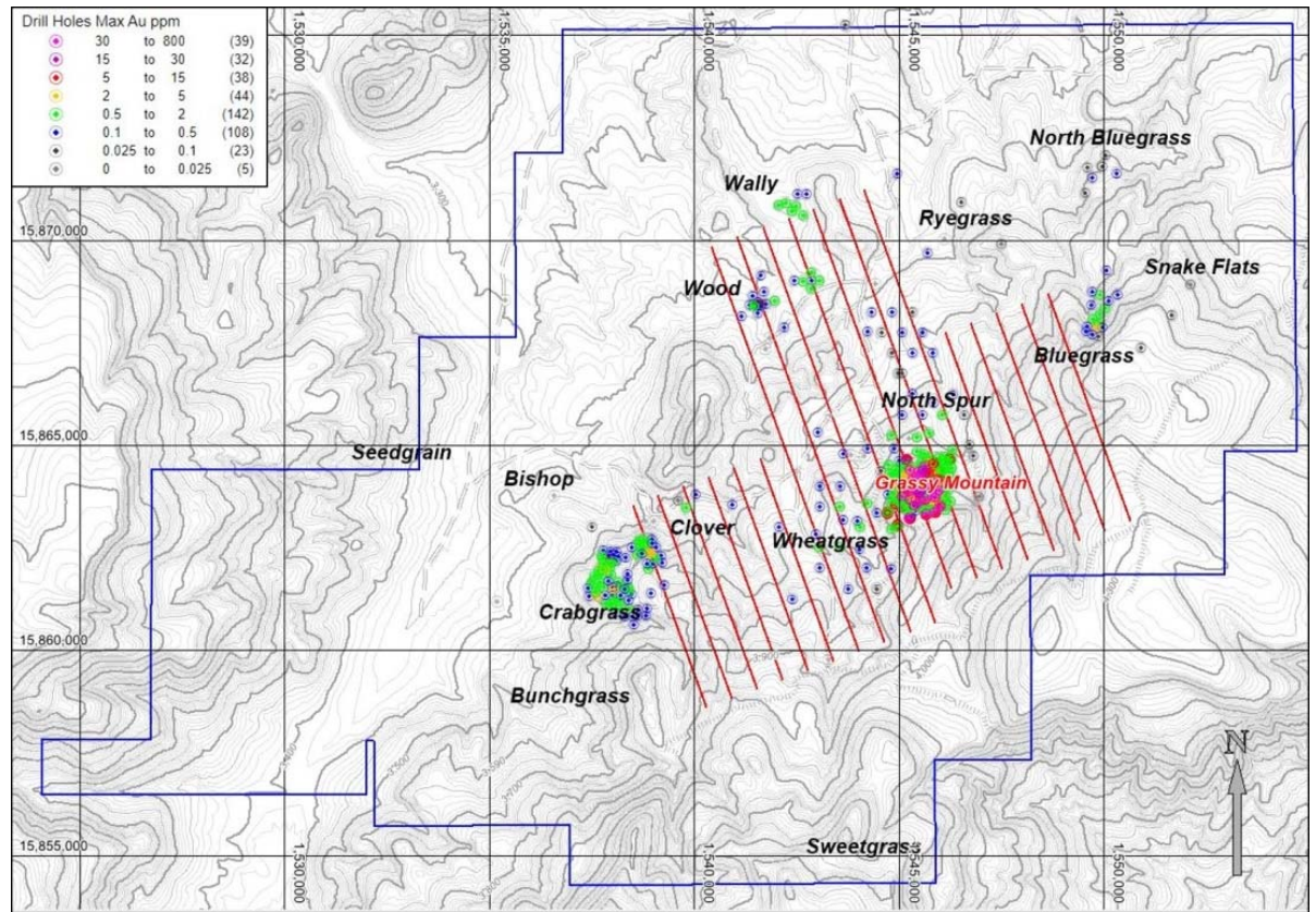
Figure 6-2: Map of 2012 CSAMT Lines
